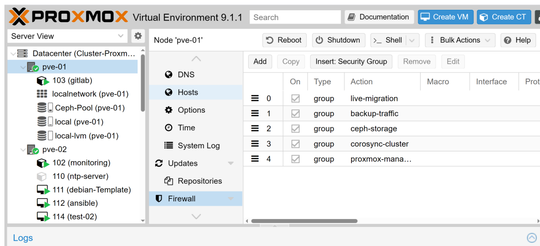
FIGURE D.4 – Règles de pare-feu configurées au niveau nœud (PVE-01) dans l'interface Proxmox (Datacenter -> pve-01 -> Firewall).
