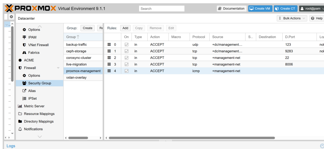
FIGURE D.3 – Groupes de sécurité configurés au niveau datacenter dans le pare-feu Proxmox.
